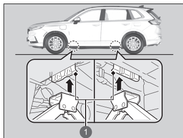
1 Puntos de apoyo para el gato
